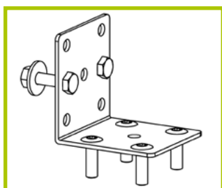
Jambages extérieurs
