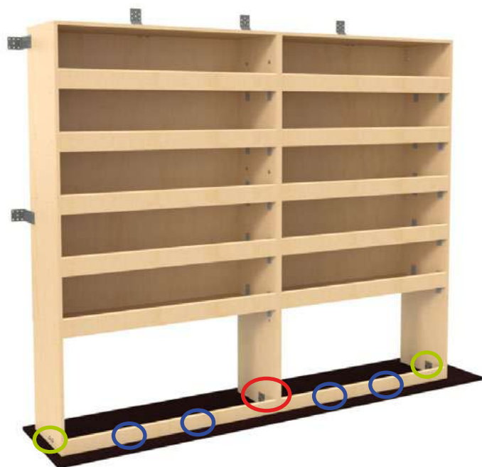
Jambages extérieurs
